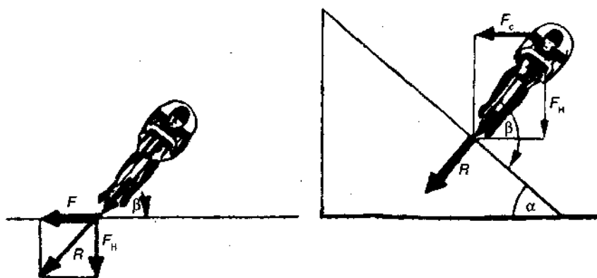
Рис. 15.39. Силы, действующие на велосипедиста при прохождении виража: F — центробежная сила, F_N — нормальная сила, R — результирующая, \alpha — угол крутизны трека, F_c — сталкивающая сила, \beta — угол наклона
