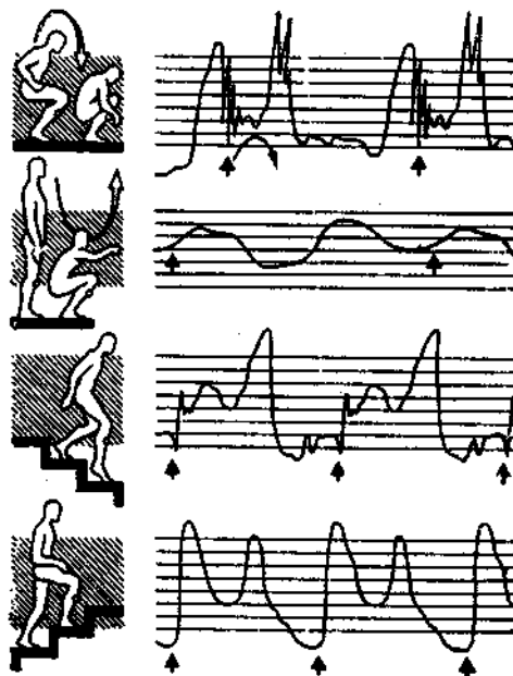
Рис. 18.35. Изгибные деформации большеберцовой кости при различных видах нагрузки
