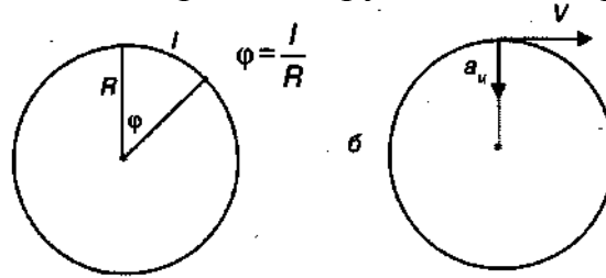
Рис. 3.19. Радианная мера угла (а). Центростремительное ускорение (б)
