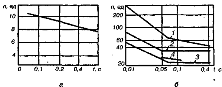
Рис. 12.1. Допустимые значения ударных перегрузок в зависимости от времени действия в направлении «таз — голова» (а) и «грудь — спина» (б): 1 — предел добровольной переносимости; 2 — выраженные физиологические реакции; 3 — слабые физиологические реакции; 4 — предел добровольной переносимости в направлении «бок — бок»
